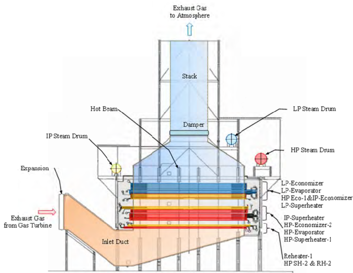
Figure 6.3.3-1 HRSG of Vertical Gas Flow Type
